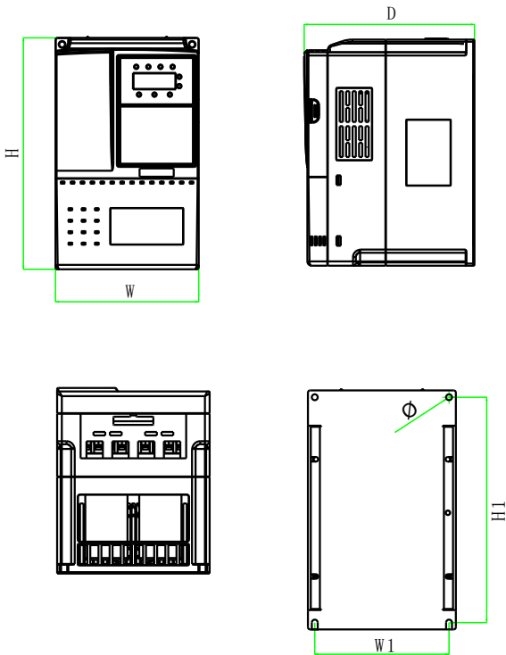
图1-1 变频器外形图
